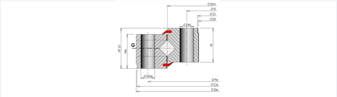
rollix-page-110-drawing.webp
