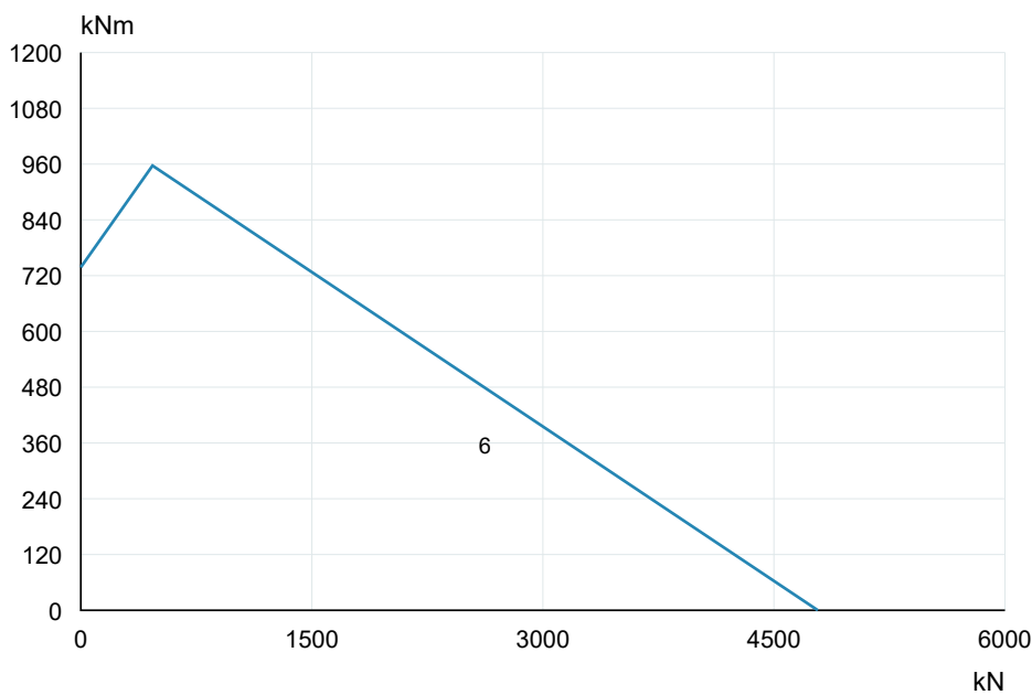
V30S021 · Curva originale 1R 6 · PDF p11
