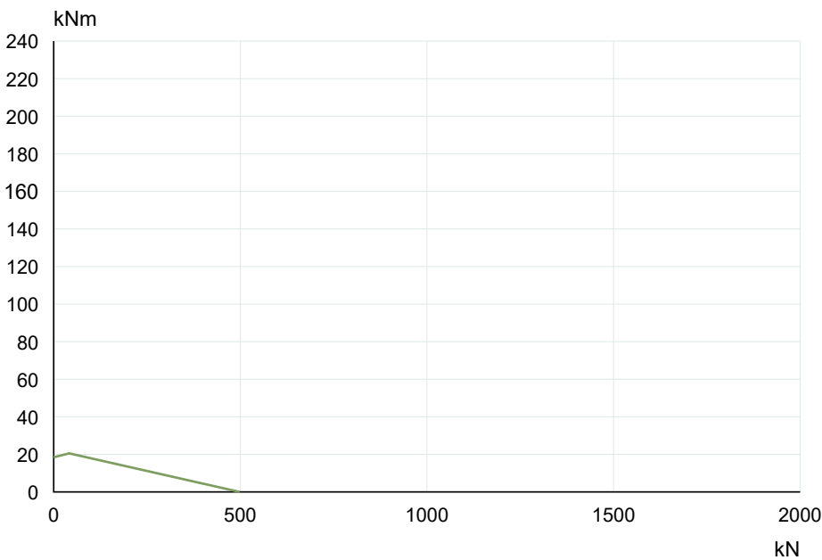
La Leonessa VE031A14 — Curva de capacidade de carga
