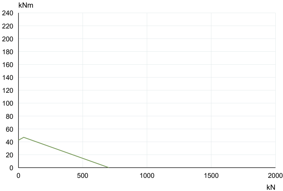
La Leonessa VE040A01 — Tragfähigkeitskurve
