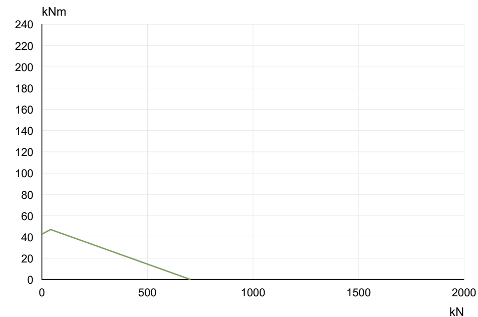
La Leonessa VE040A01 — Curva de capacidad de carga
