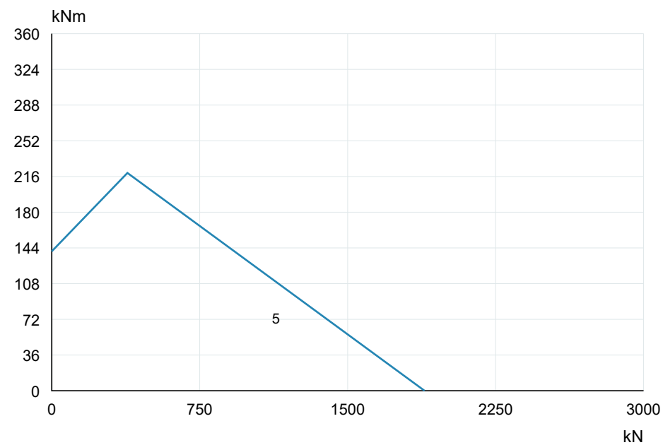
VE061B05 · Curva original 2SE 5 · PDF p7
