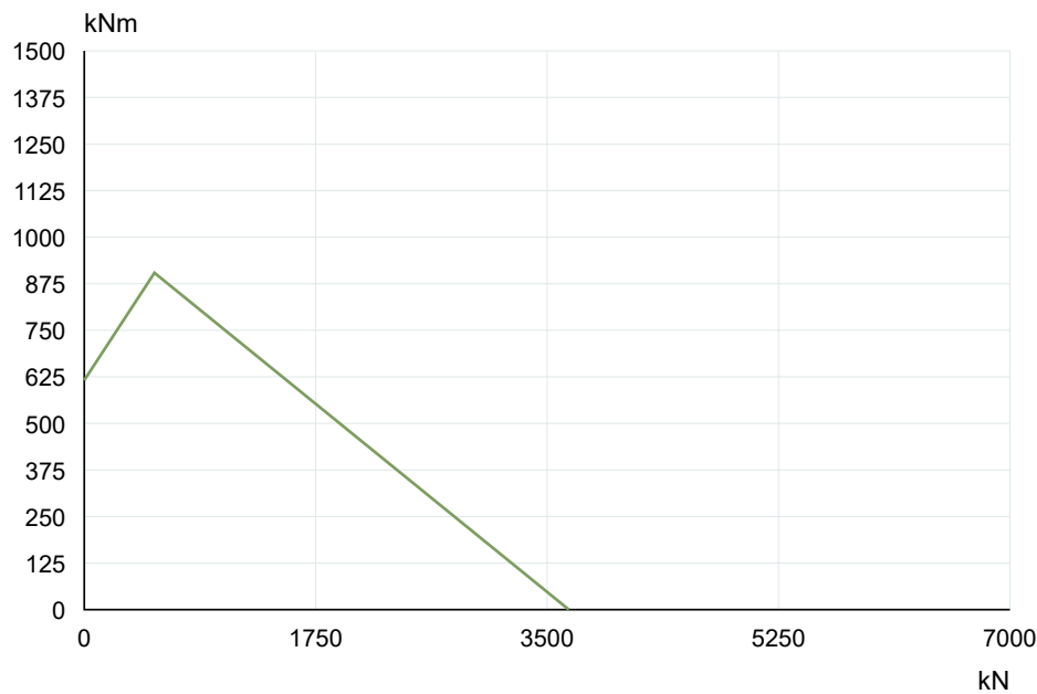
La Leonessa VE140A01 — Tragfähigkeitskurve
