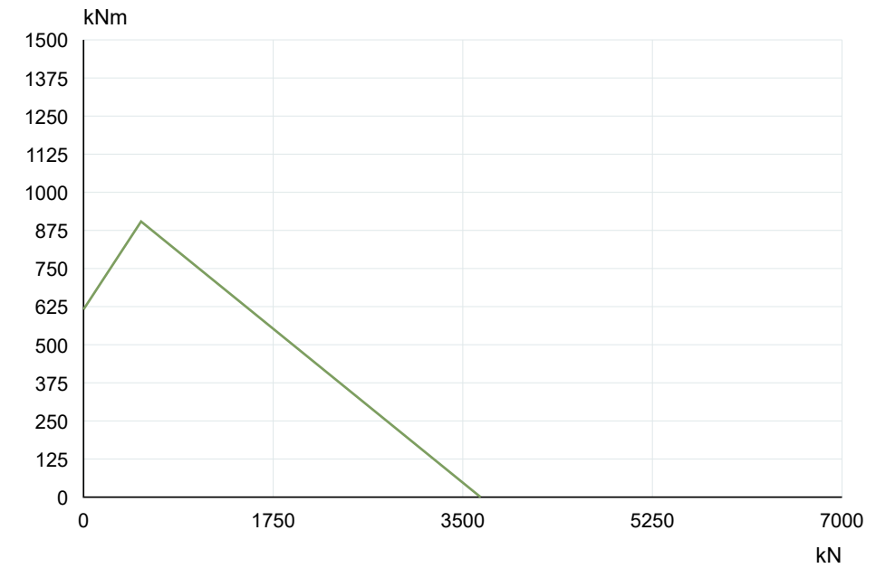
La Leonessa VE140A01 — Curva de capacidade de carga
