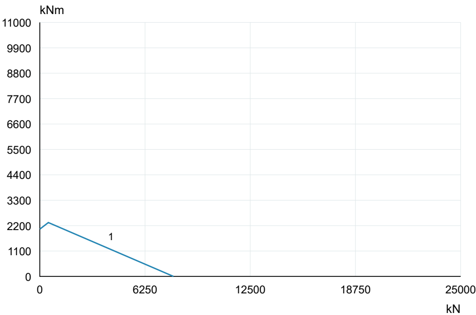
VE160B00 · Curva originale 2SE 1 · PDF p15
