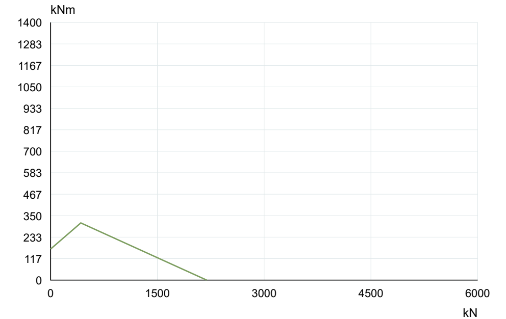
La Leonessa VI085A05 — Curva di capacità di carico
