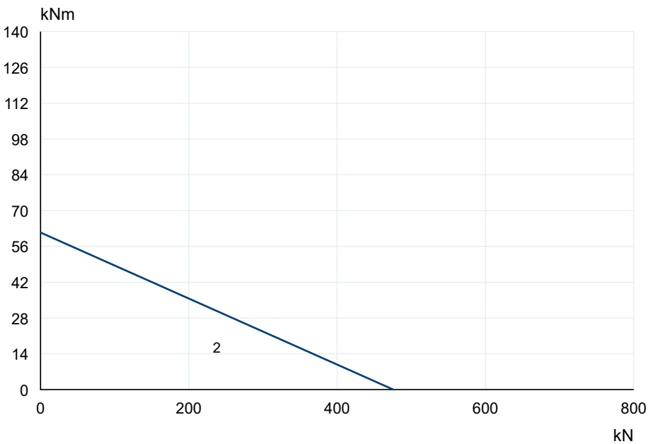
VS070UE00 · Исходная кривая U 2 · PDF стр. 6
