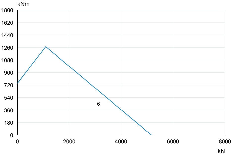
VS147B00 · Curva originale 2S 6 · PDF p11
