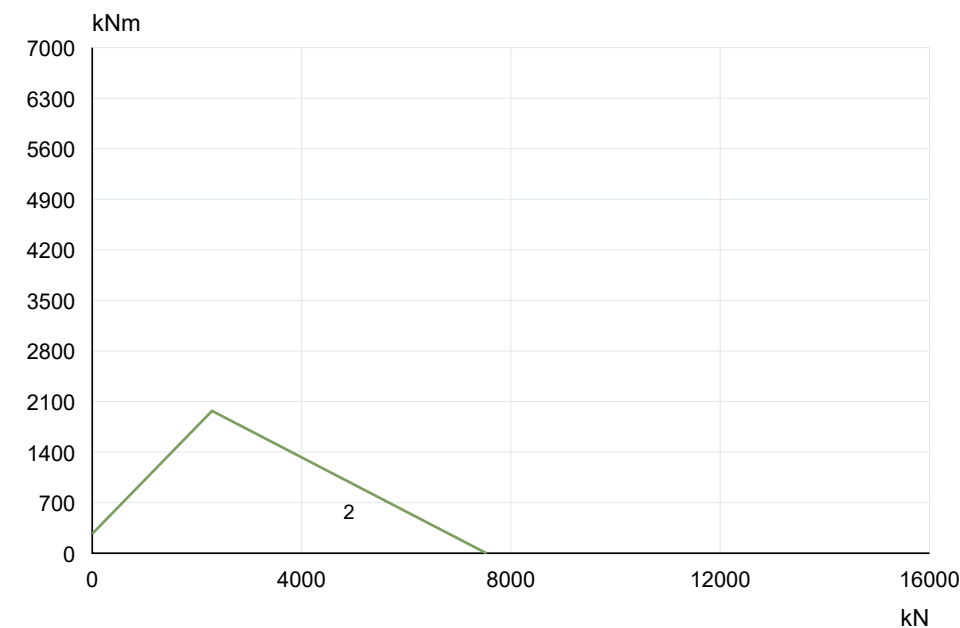
VS171A00 · Исходная кривая 1S 2 · PDF стр. 24
